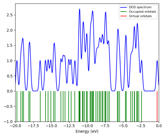
Fig. 7: UV-Vis Spectra and DOS
