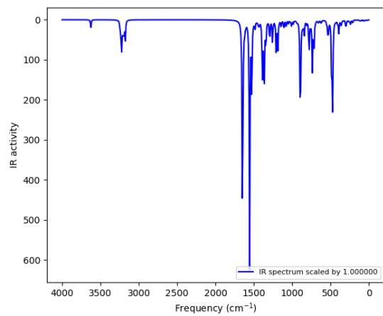
Fig. 5: IR Spectra
