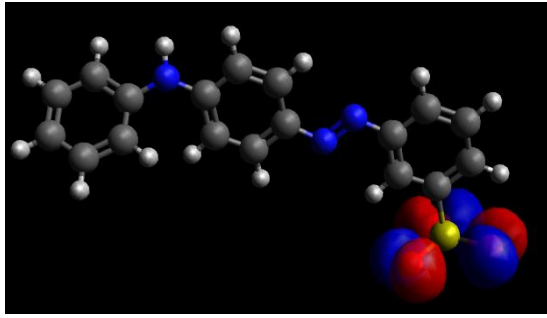
Fig. 3.1: HOMO
