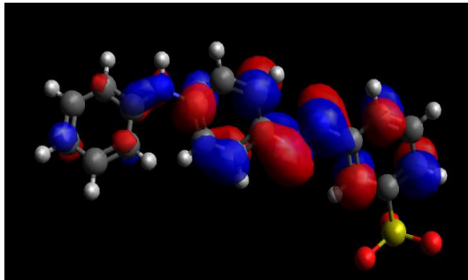
Fig. 3.2: LUMO
