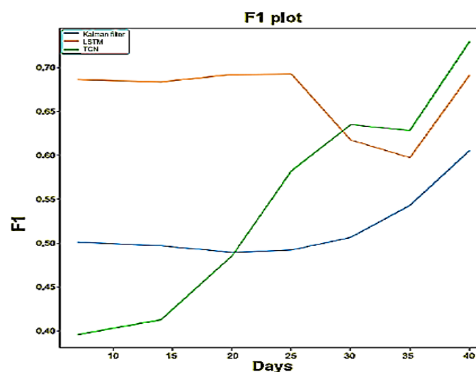
Fig. 23: F1 plot
