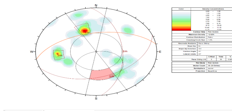
Fig. 12: Planar Failure Criteria.
